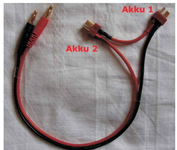
Wichtig Immer zuerst Akku 1 dann 2 dann 3 anschließen
